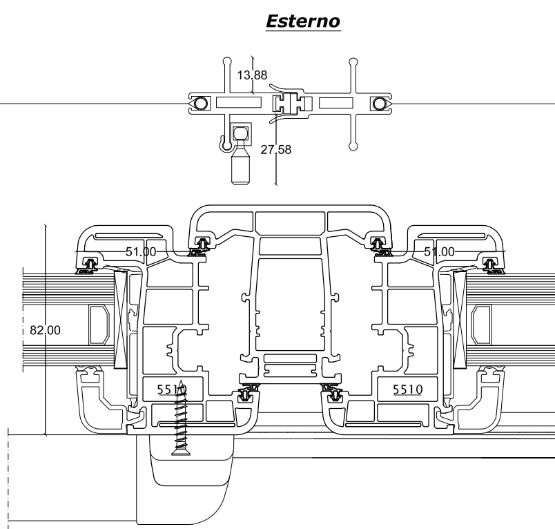
Sezione B - orizzontale
