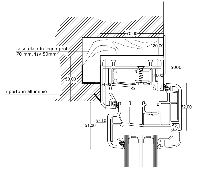
Sezione A - verticale
