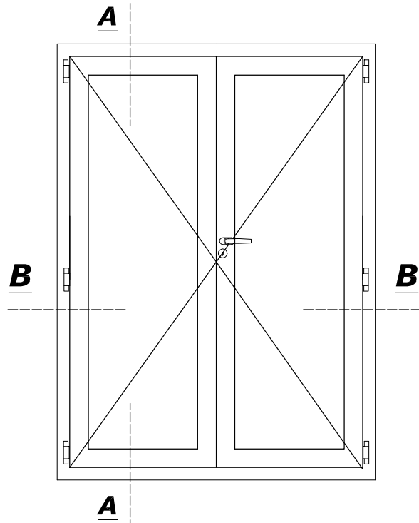
Prospetto - Fuori scala
