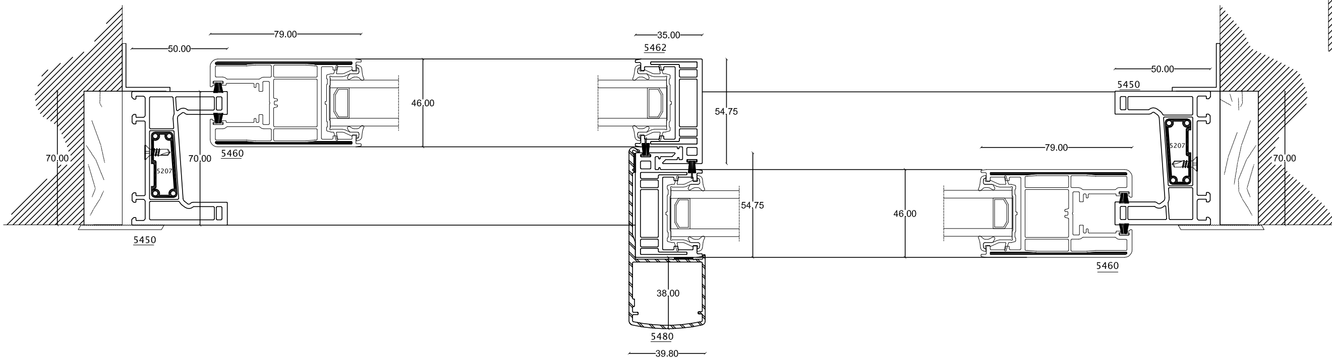
Sezione B - orizzontale
