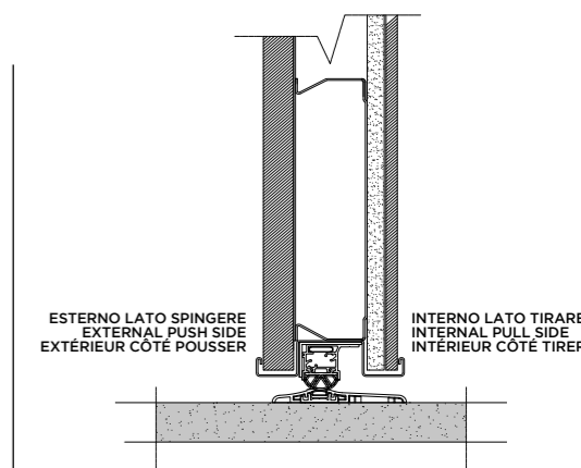
SOGLIA PER KIT ARIA - ACQUA - VENTO Aev Kit Seuil pour kit AEV
